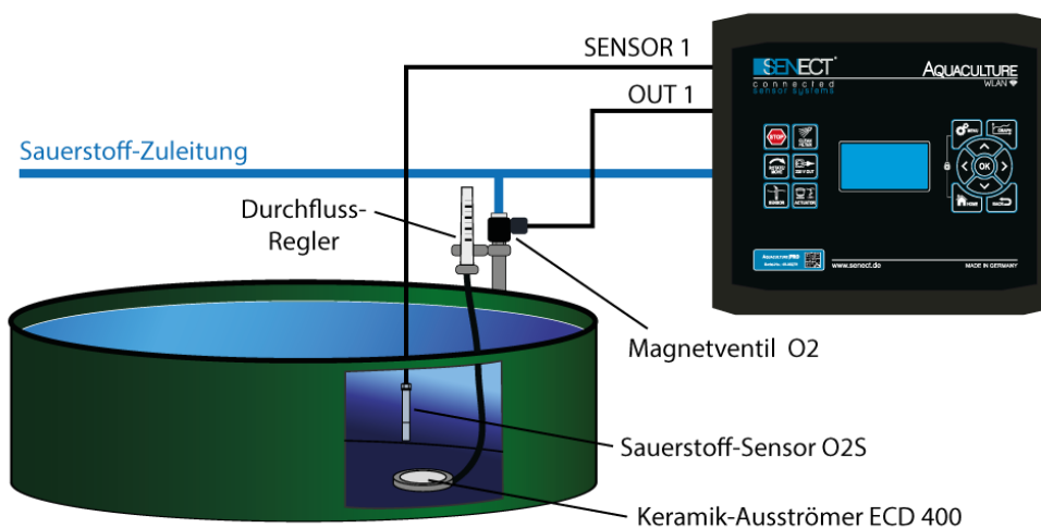
Abbildung 4: Anschlussbeispiel Sauerstoffregelung.
